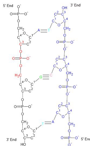
Cấu trúc xoắn kép của DNA (DeoxyriboNucleic Acid) { https://en.wikipedia.org/wiki/Francis_Crick }
